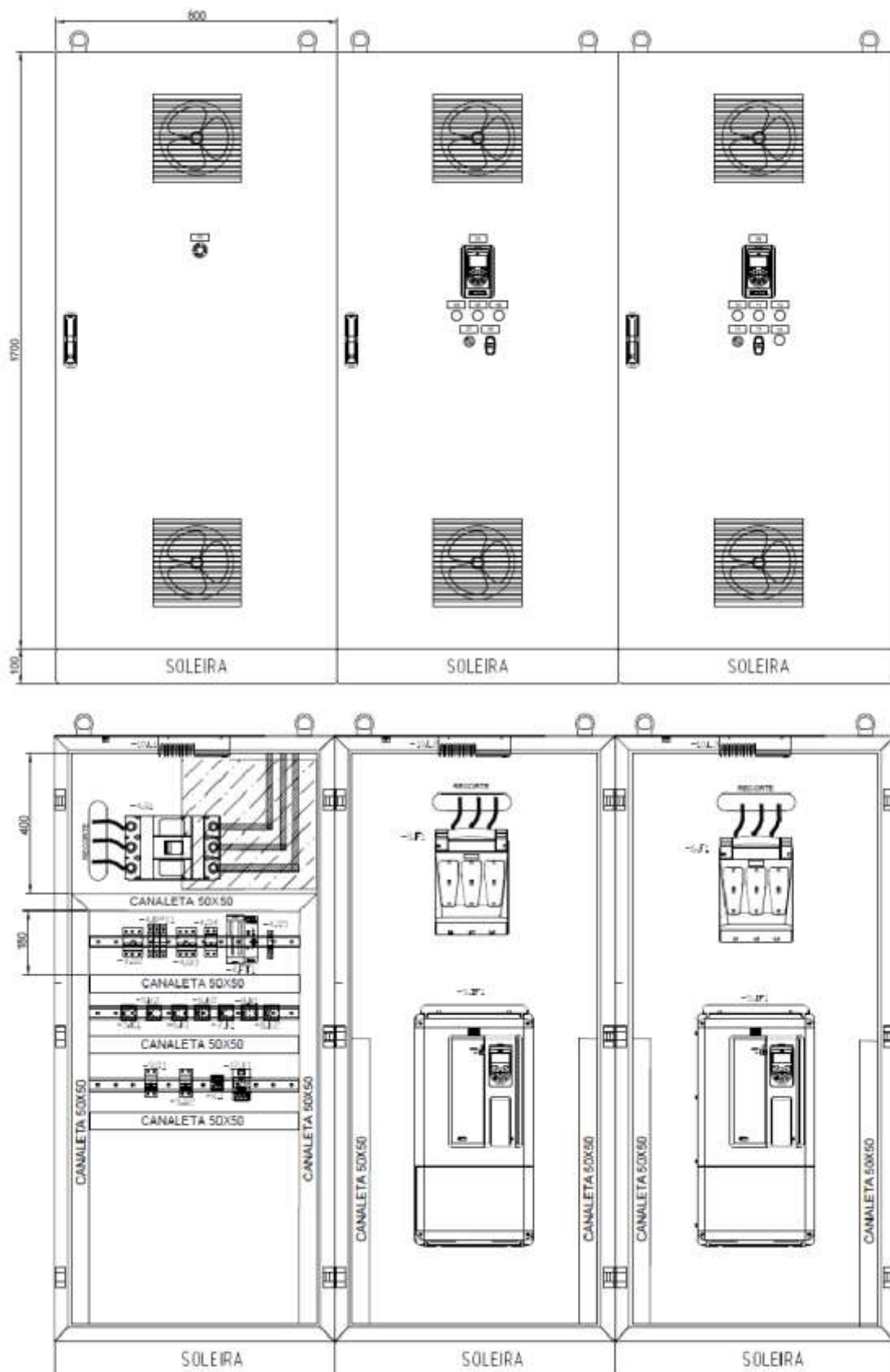
Figura 1: Layout de montagem orientativo do painel poço profundo UC5 – Barro Preto.
